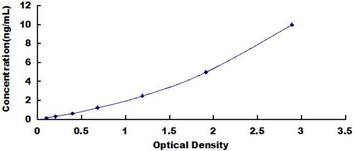
大鼠 S100 钙结合蛋白 A8 (S100A8) 检测试剂盒标准曲线
